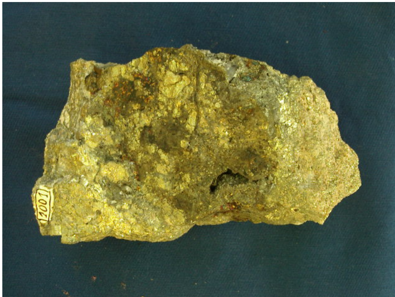
1001 - Pirita arsenopirita e calcopirita - Potosi - Bolívia
