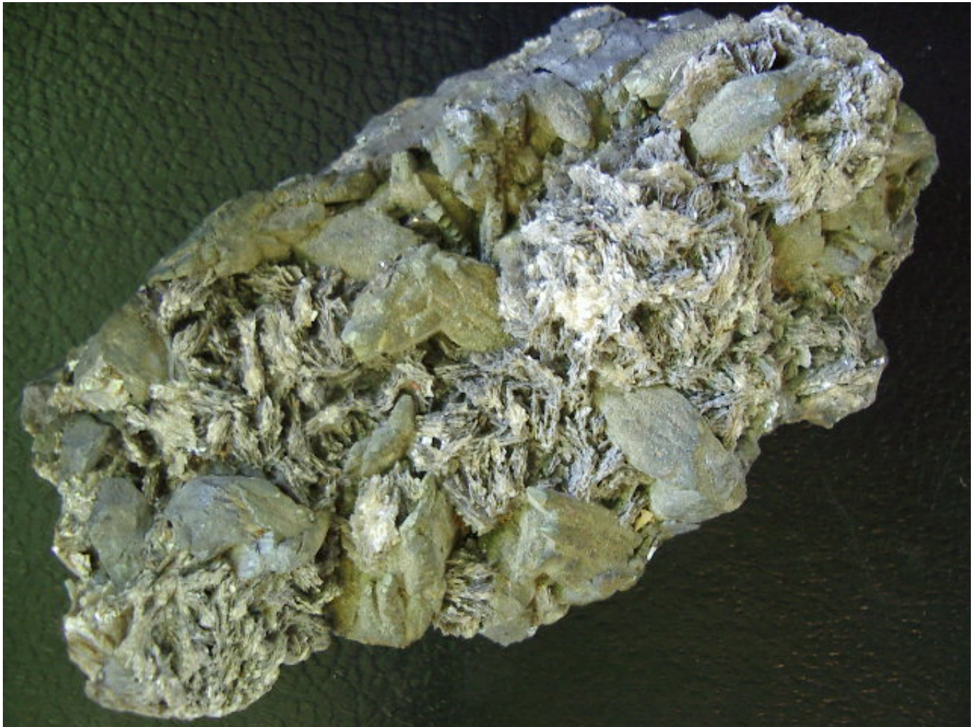
957 - Arsenopirita muscovita e marcassita
