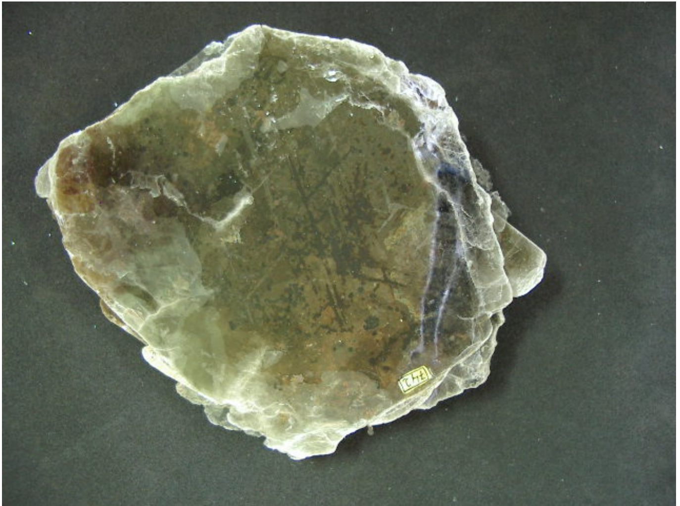
742 - Muscovita - Procedência desconhecida
