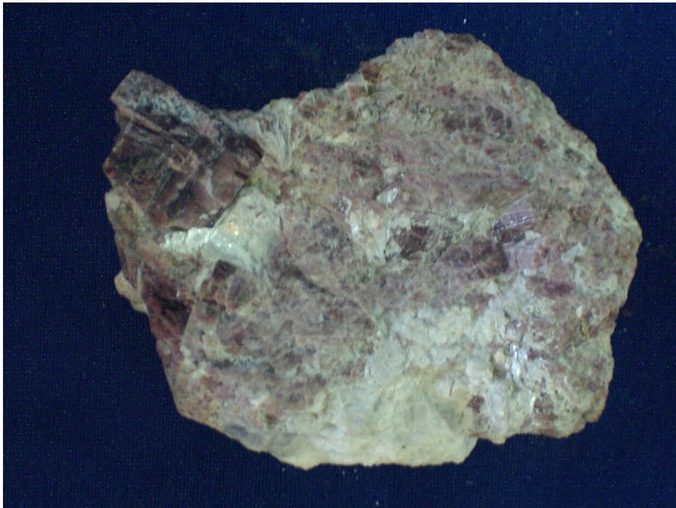
600 - Rubelita albita e muscovita - Araçuaí MG
