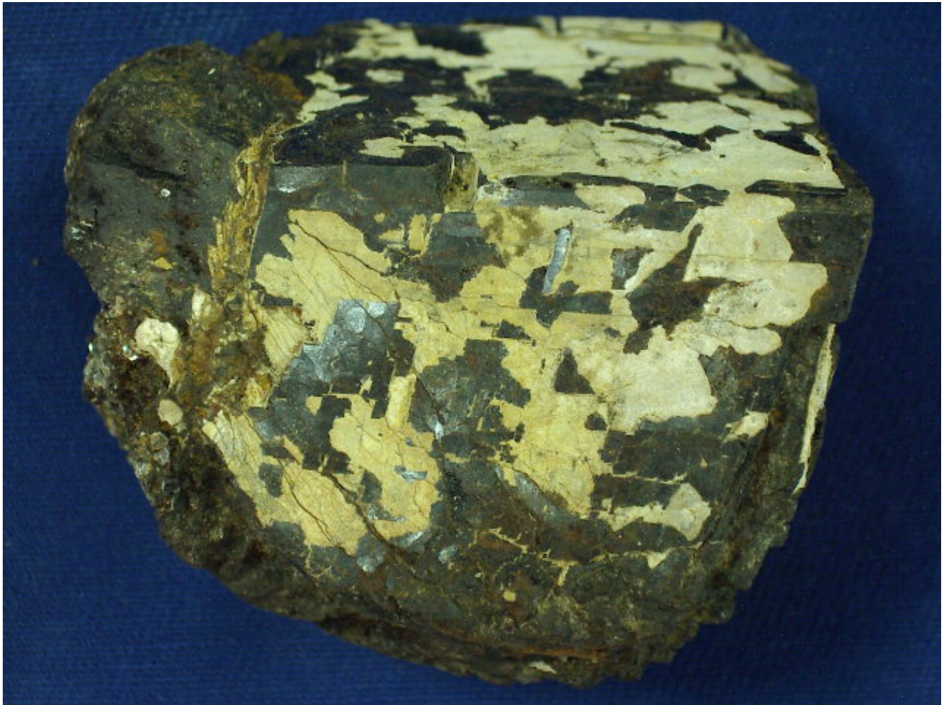
317 - Goethita e hematita - Fábrica Nacional de Motores RJ
